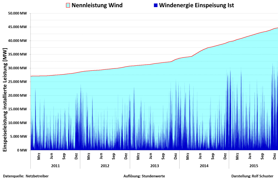
Installierte Leistung versus tatsächliche Einspeisung, Darstellung durch Rolf Schuster. Daten: EEX.
